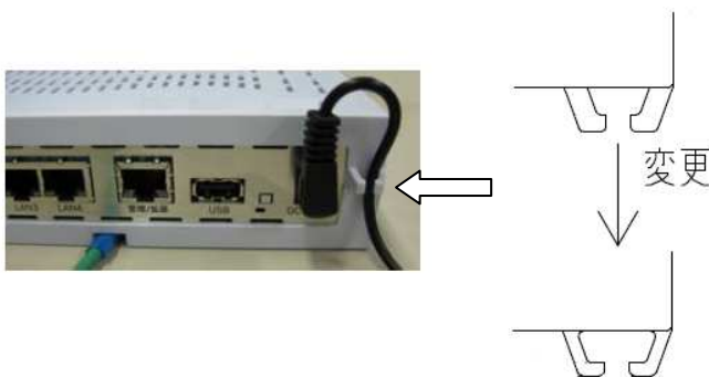
図1 電源コード用クランプ部変更
